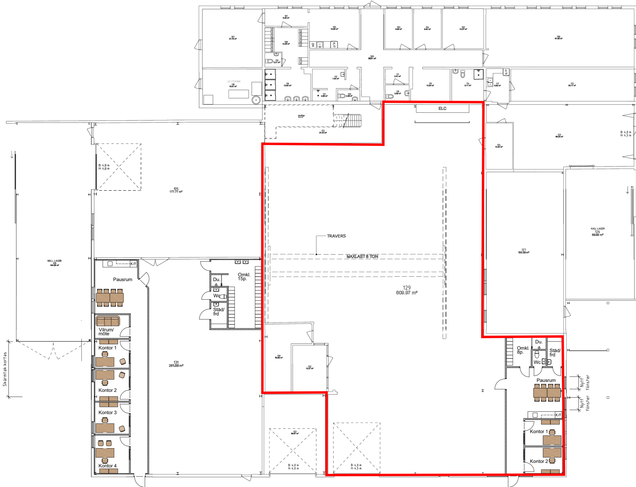
PLAN 1, ÖVERSIKTSRITNING OMBYGGNAD SKALA 1:100 (A1)
