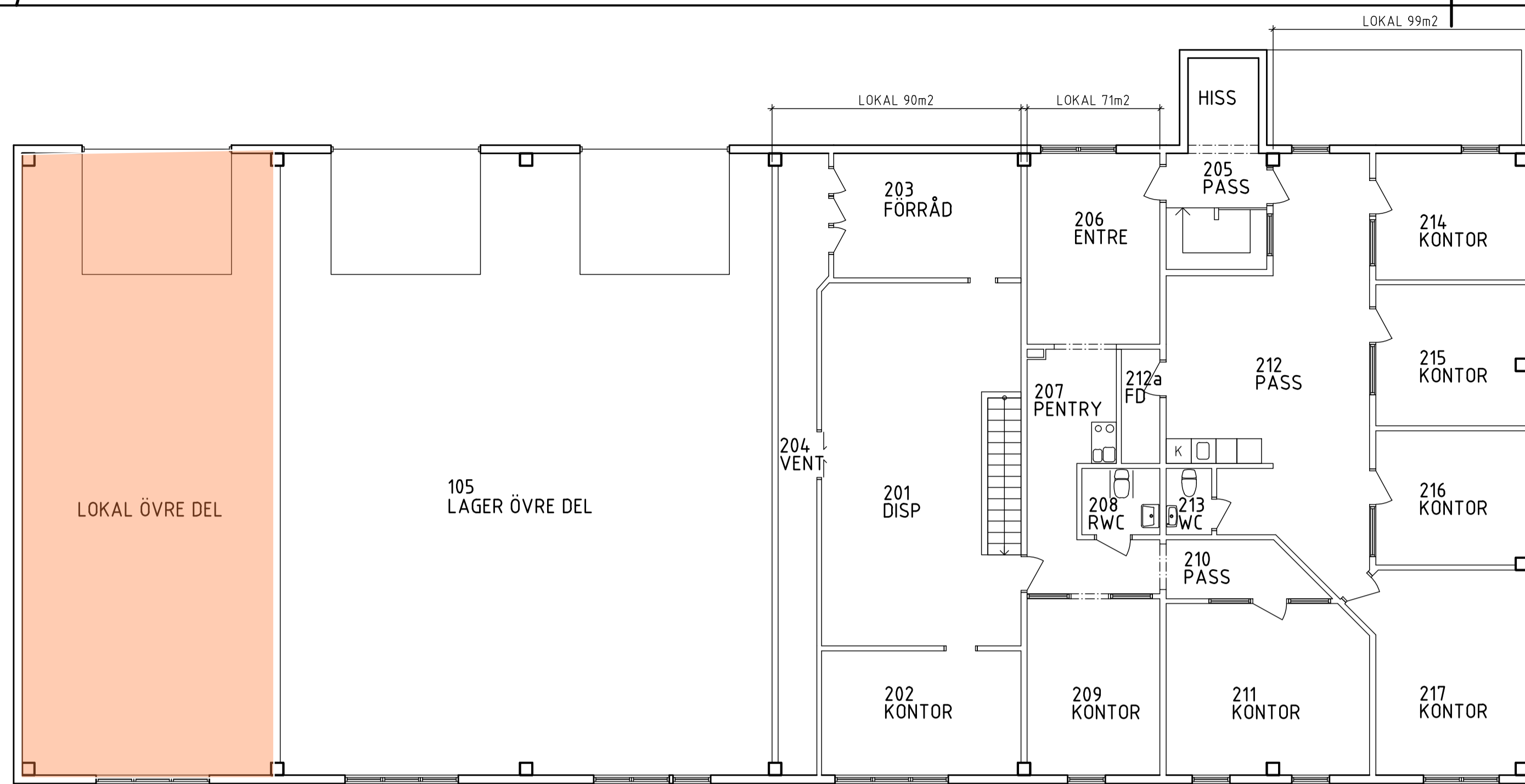
PLAN 1 TR. - 1:100
